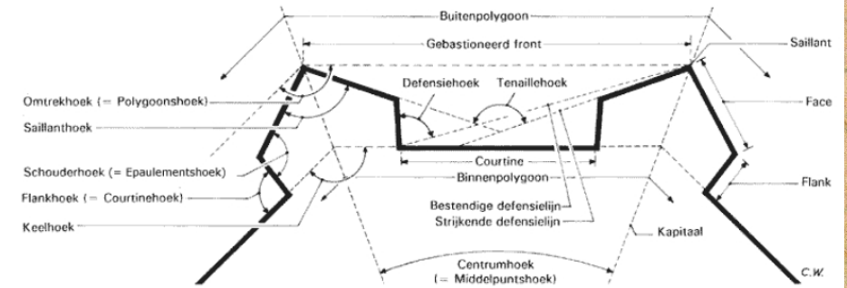
CONSTRUCTIELIJNEN en -HOEKEN v e GEBASTIONEERD TRACE
