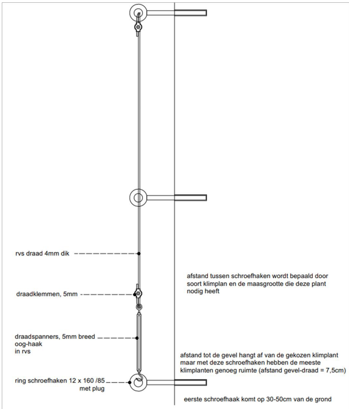
Figuur 1: schematische voorstelling hoe klimhulp te bevestigen aan de muur
