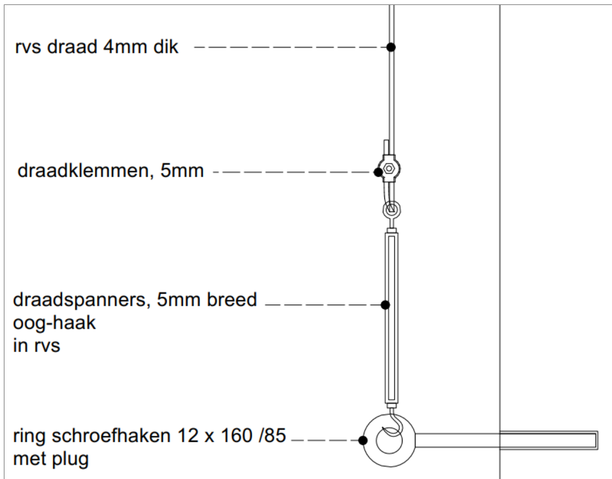
Figuur 2: detail schema bevestiging klimhulp
